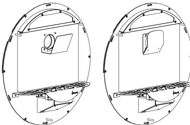
REDUZIERSTÜCK A
