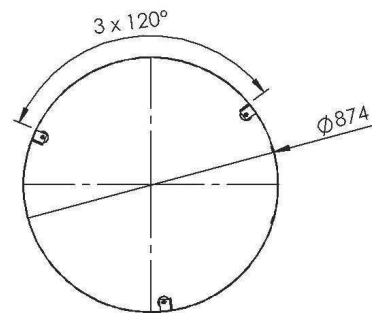
COUPE A-A
